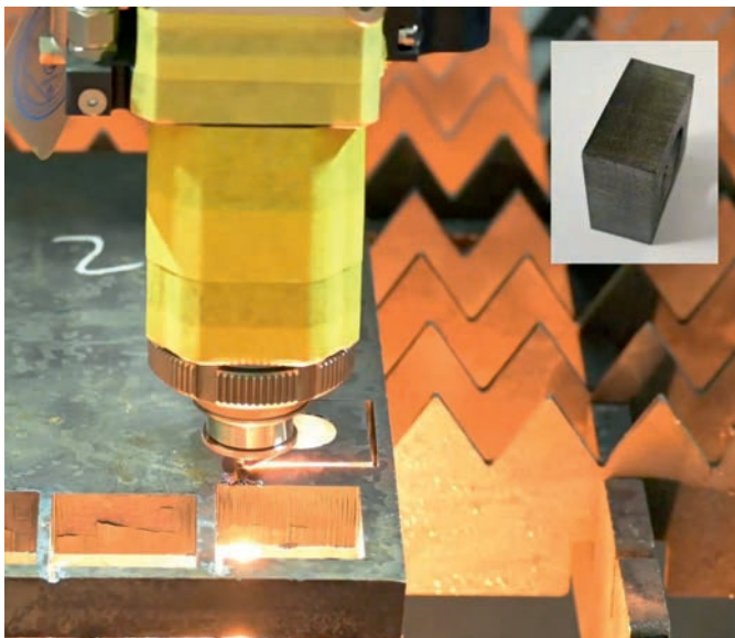
Dickblechschneiden (6kW)
